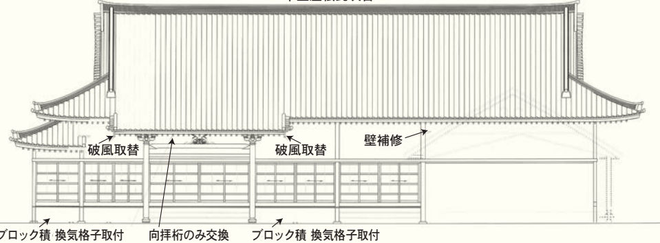
本堂大屋根大改修完成予定図
